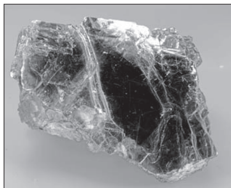
Muskovit, Norsko.
