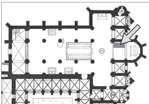
Umístění rožmberské hrobky v presbytáři kostela Nanebevzetí Panny Marie ve Vyšším Brodě, zaměření Jiří Šindelář.
